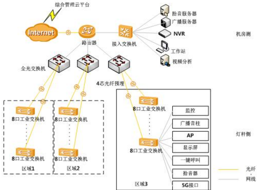
智慧灯杆组网拓扑图
