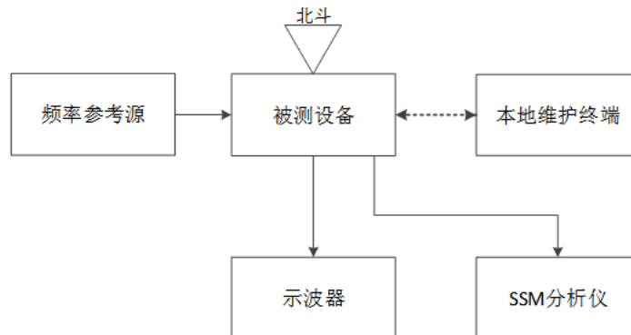
图 3 频率输出功能测试配置图
