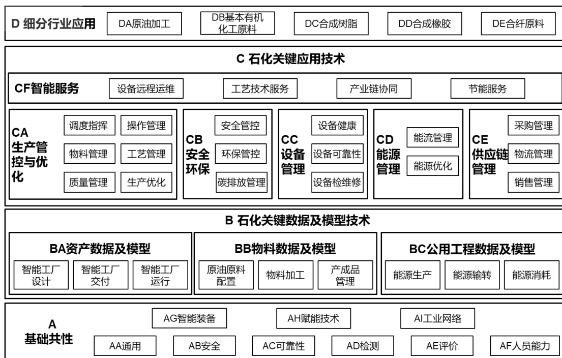
图 1 石化行业智能制造标准体系结构图
